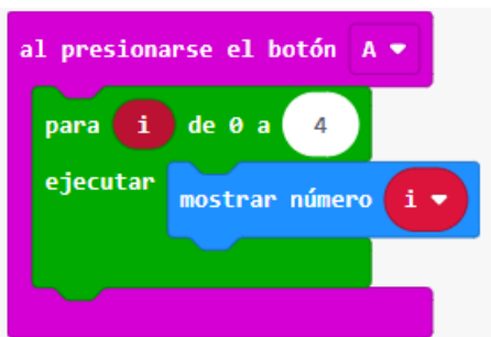
Figura 1 – Ejemplo del uso del ciclo “para”
