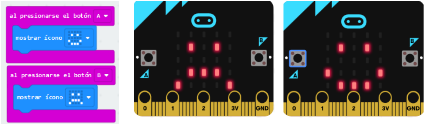
Figura 4 - Algoritmo desarrollo y resultados obtenidos para el ejemplo 2
