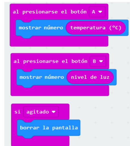
Figura 5 - Algoritmo del ejemplo 3
